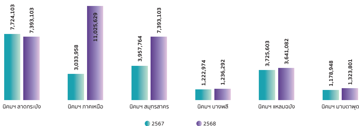
ปริมาณน้ำดิบ นิคมฯ มาบตาพุด เปรียบเทียบ ปี 2567 - 2568
