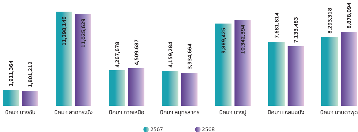
ปริมาณน้ำเสียที่บำบัด (ลบ.ม.) ตามสัญญา OMA เปรียบเทียบ ปี 2567 - 2568
