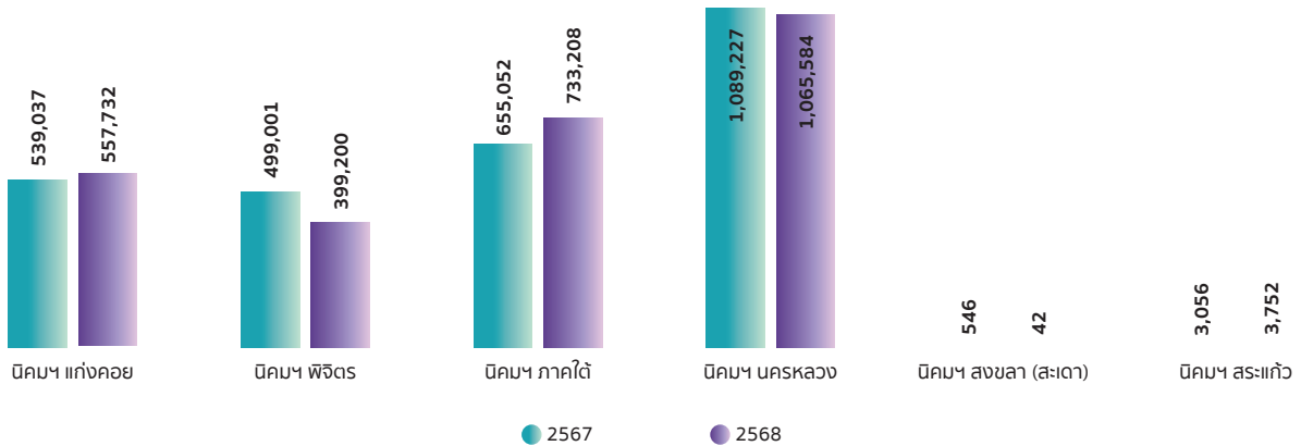
ปริมาณน้ำเสียที่บำบัด (ลบ.ม.) ตามสัญญา O&M เปรียบเทียบ ปี 2567 - 2568
