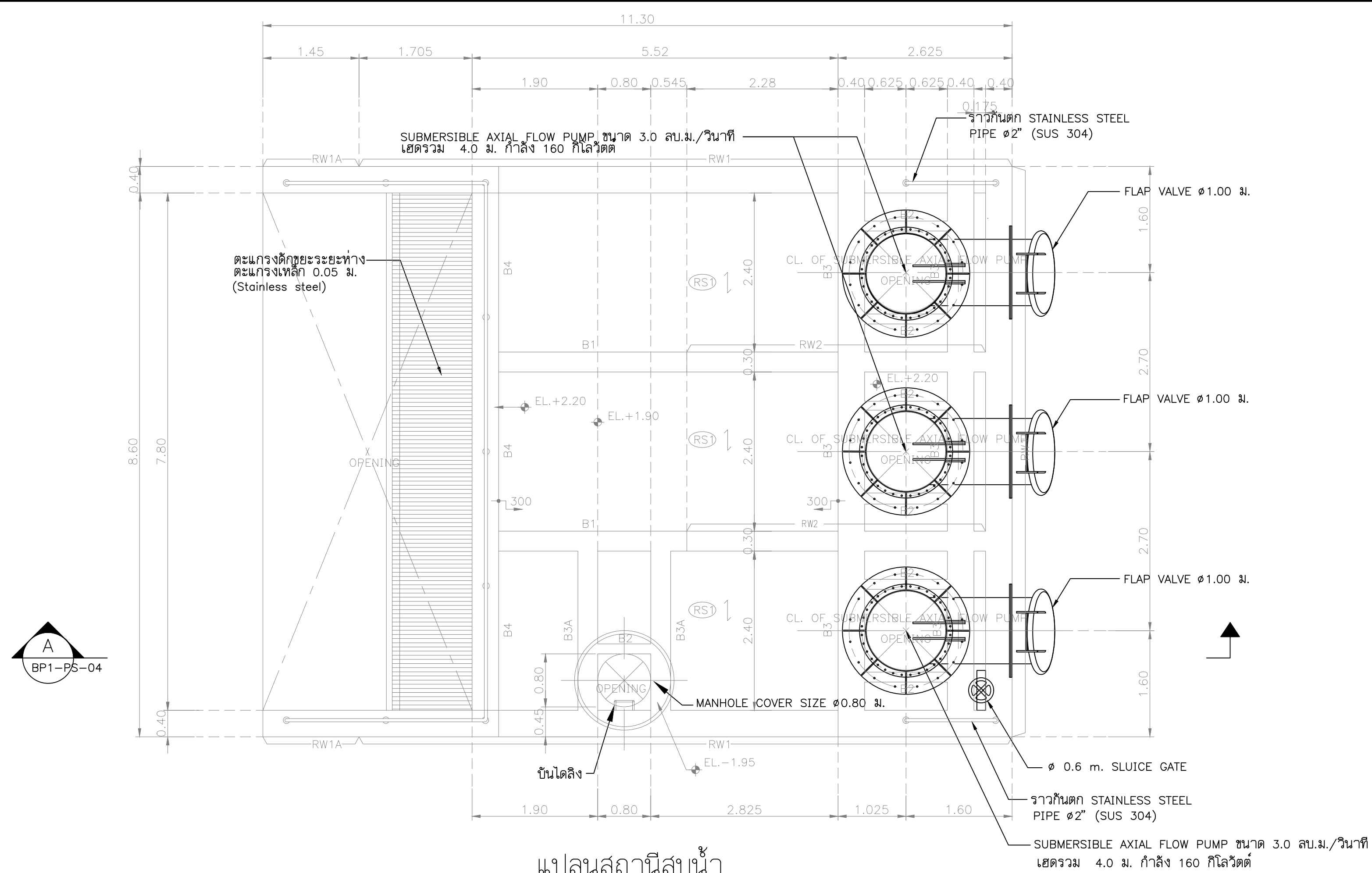
แปลนสถานีสูบน้ำ SCALE 1:50
