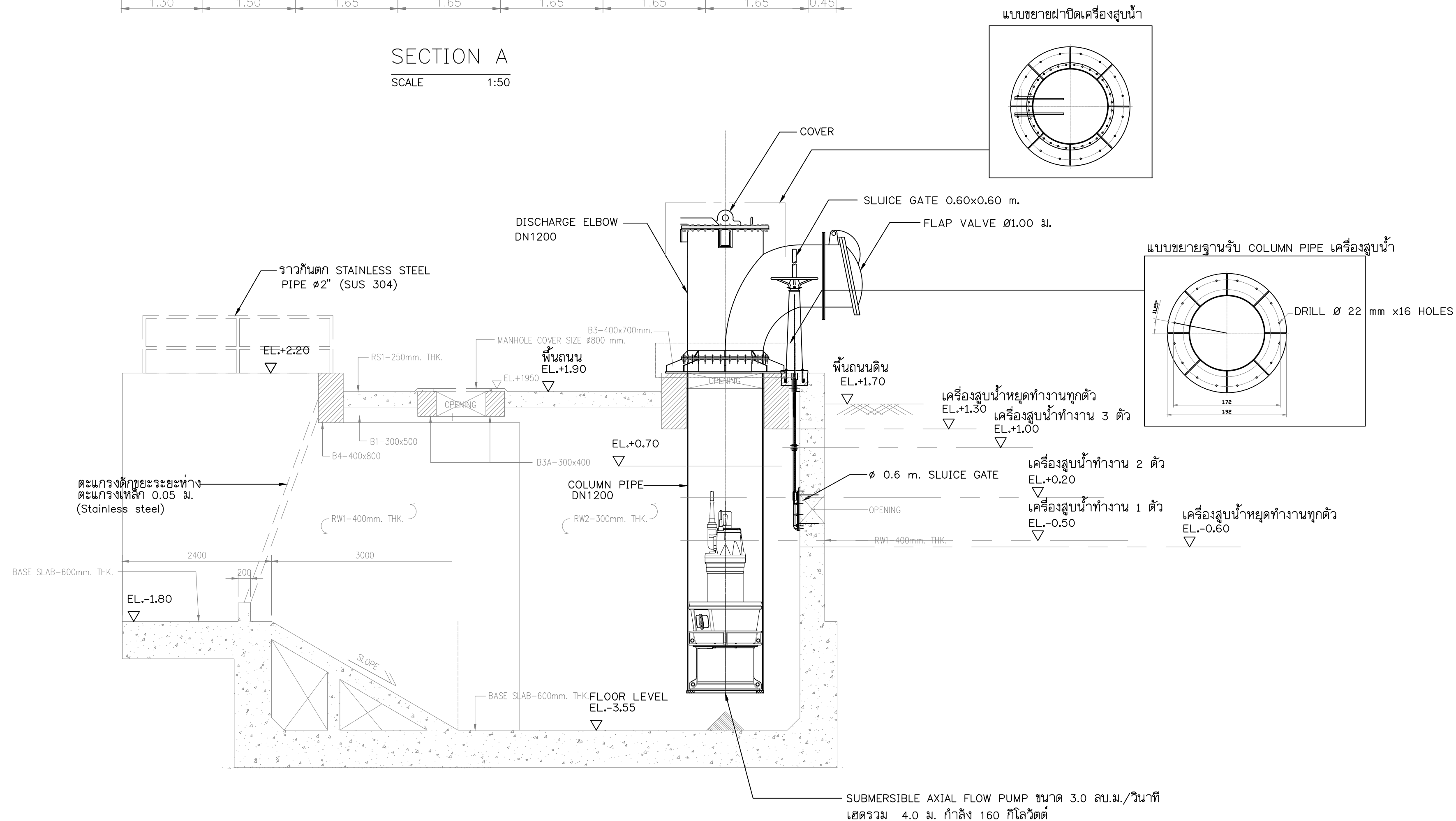
แบบแสดงรายละเอียดและค่าระดับน้ำทำงานของเครื่องสูบน้ำ SCALE 1:50
