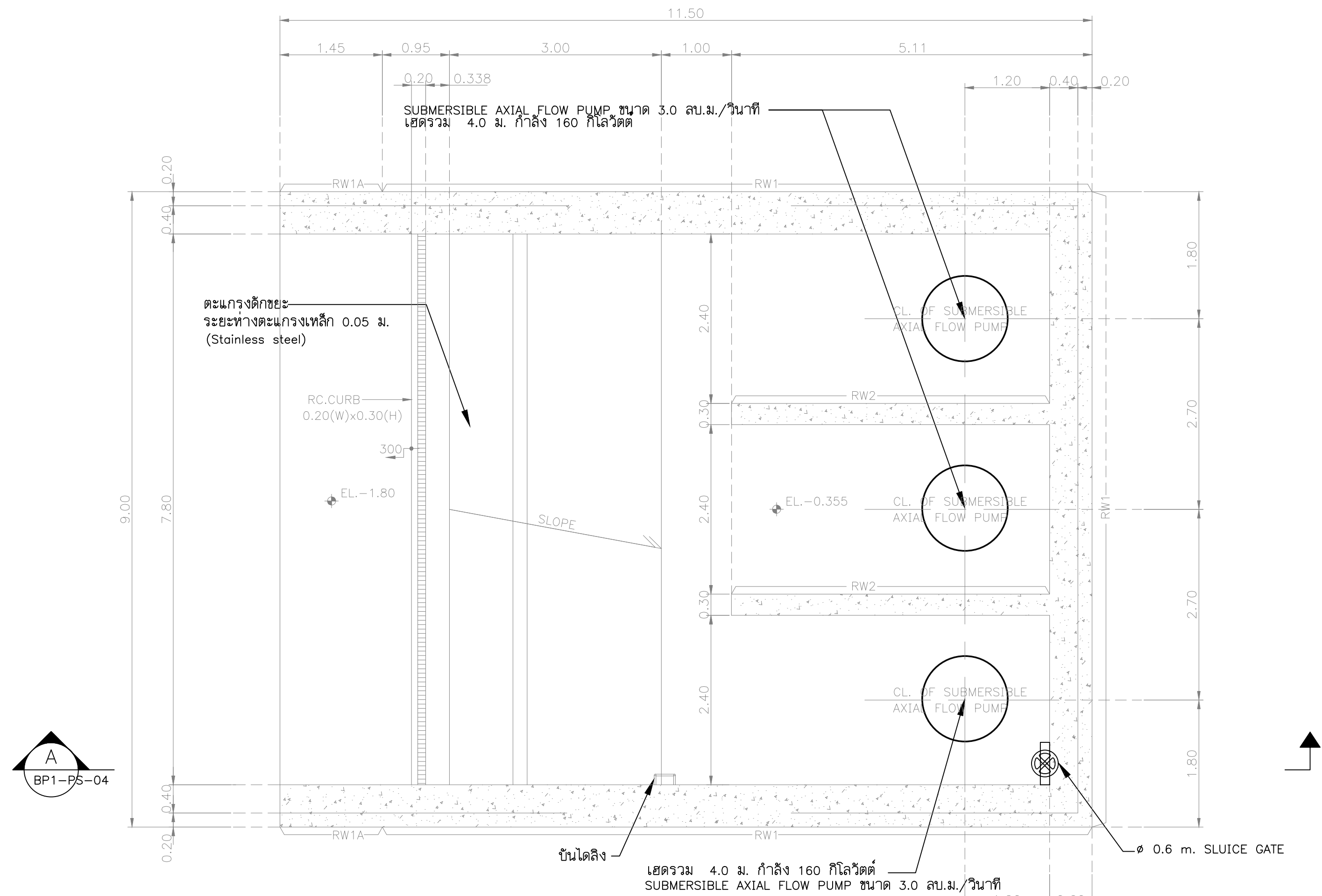
รูปตัดแปลนสถานีสูบน้ำ SCALE 1:50
