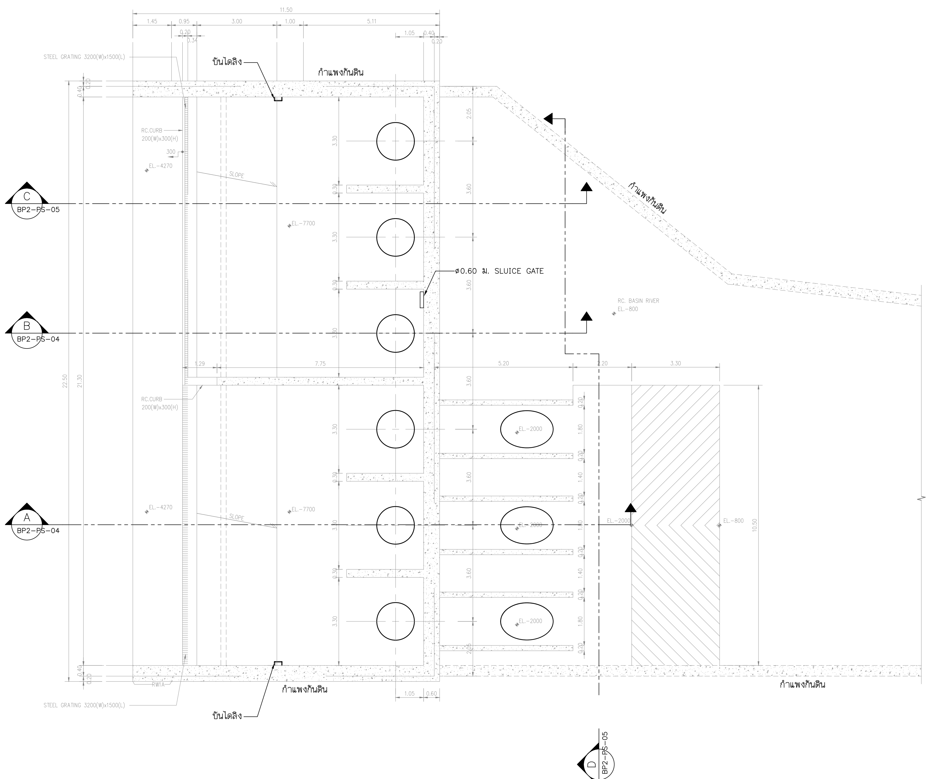
แปลนสถานีสูบน้ำที่ระดับ -0.80 ม.รทก. SCALE 1:75
