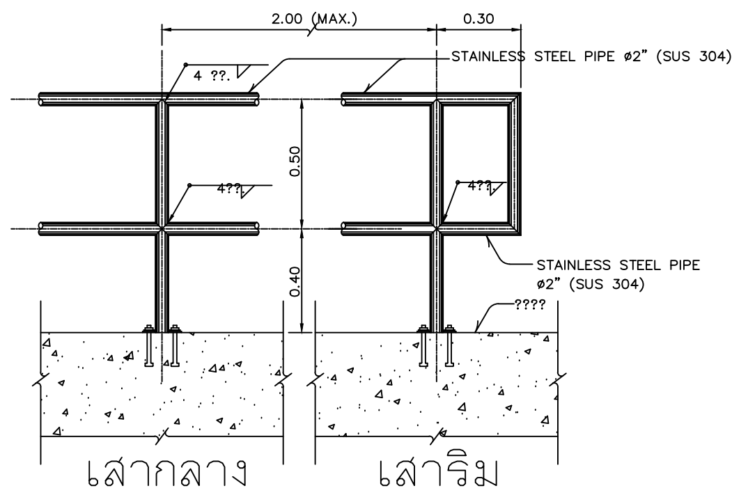
แบบขยายราวกันตก ไม่แสดงมาตราส่วน
