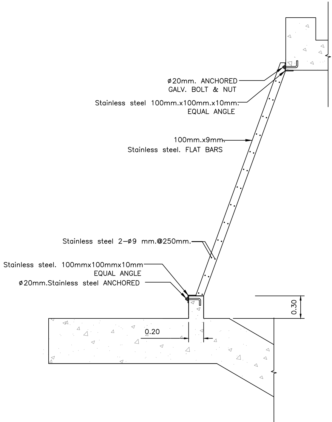
รายละเอียดฐานรองรับตะแกรงเหล็กดักขยะ ไม่แสดงมาตราส่วน
