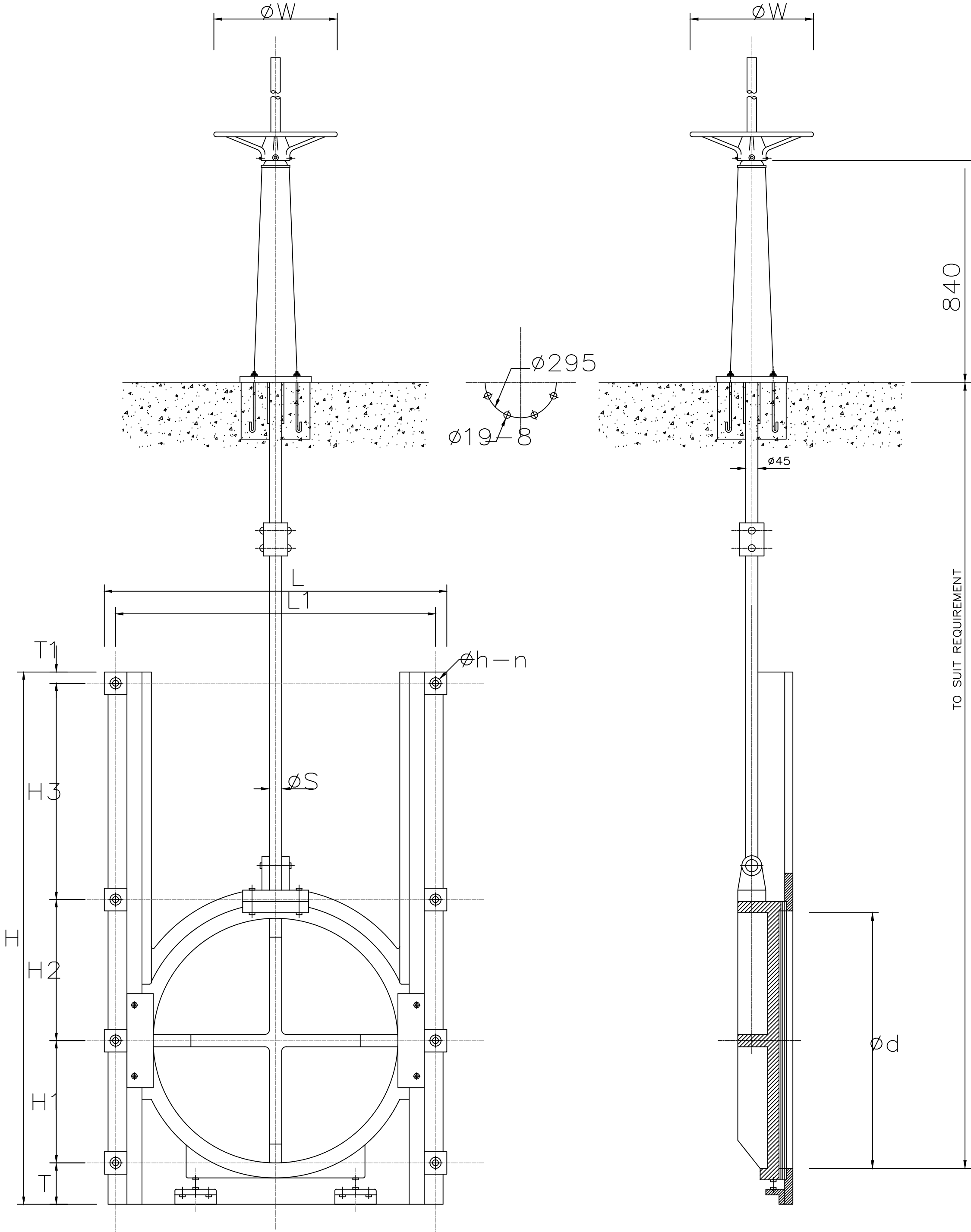
รูปด้านหน้าและรูปด้านข้างบานฝาท่อ ขนาด ๑600 mm. ไม่แสดงมาตราส่วน
