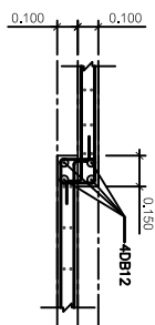
แบบขยายกรณีเปลี่ยนระดับพื้น SCALE 1:20
