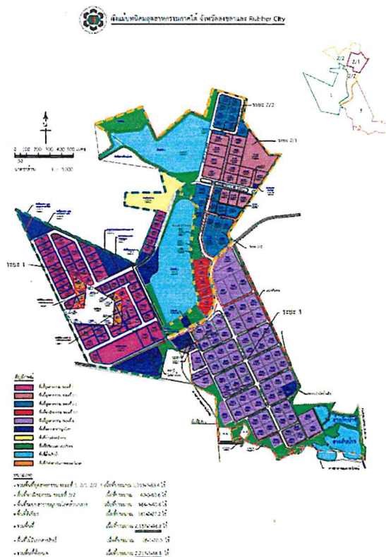
รูปที่ 1 ผังการใช้ประโยชน์ที่ดินของนิคมอุตสาหกรรมภาคใต้ จังหวัดสงขลา
