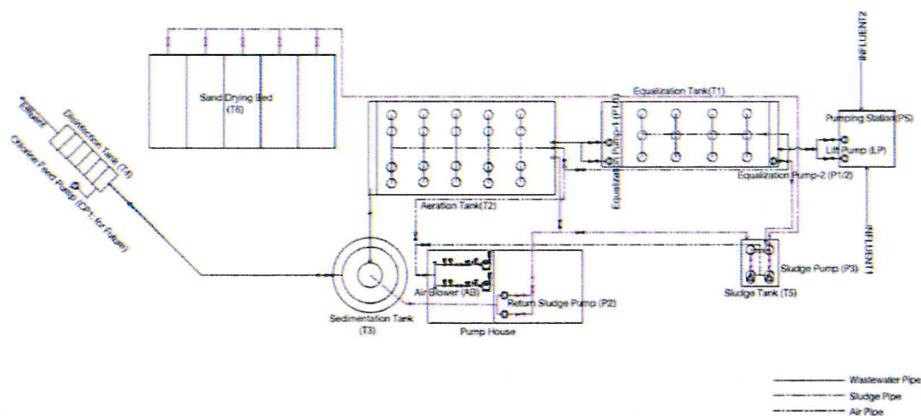
รูปที่ 1 Layout ระบบบำบัดน้ำเสียสำนักงานท่าเรืออุตสาหกรรมมาบตาพุด
