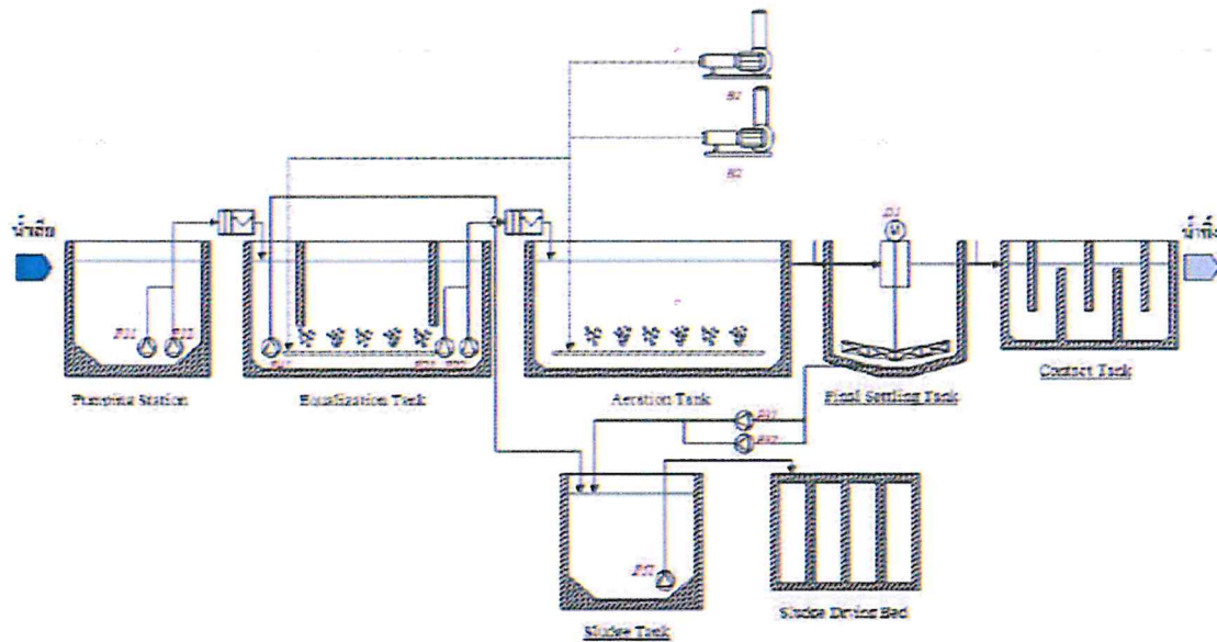
รูปที่ 2 ผังการไหลของระบบบำบัดน้ำเสียสำนักงานท่าเรืออุตสาหกรรมมาบตาพุด
