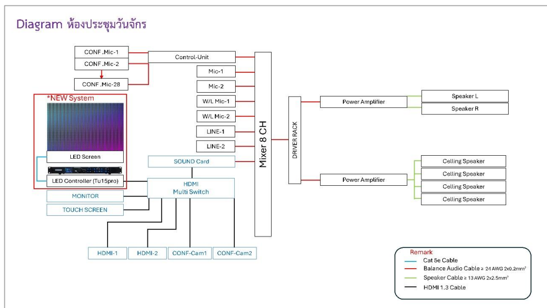
รูป 5.2 - ไดอะแกรมติดตั้งระบบภาพและเสียง ห้องประชุมวันจักร
