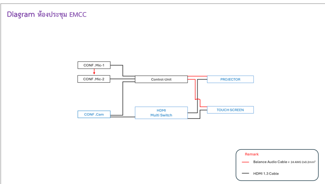
รูป 3.2 - ไดอะแกรมติดตั้งระบบภาพและเสียง ห้องประชุม EMCC
