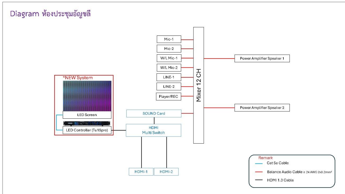
รูป 9.2 - ไดอะแกรมติดตั้งระบบภาพและเสียง ห้องประชุมอัญชลี
