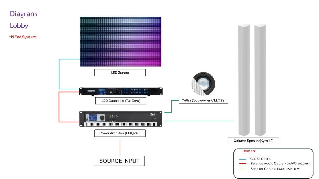
รูป 1.1 - ไดอะแกรมติดตั้งระบบภาพและเสียง ห้องโถงชั้น 1
