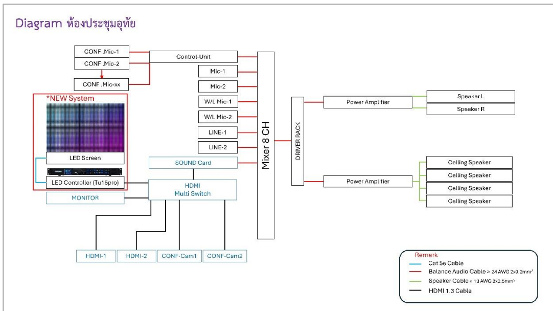
รูป 4.2 - ไดอะแกรมติดตั้งระบบภาพและเสียง ห้องประชุมอูทัย
