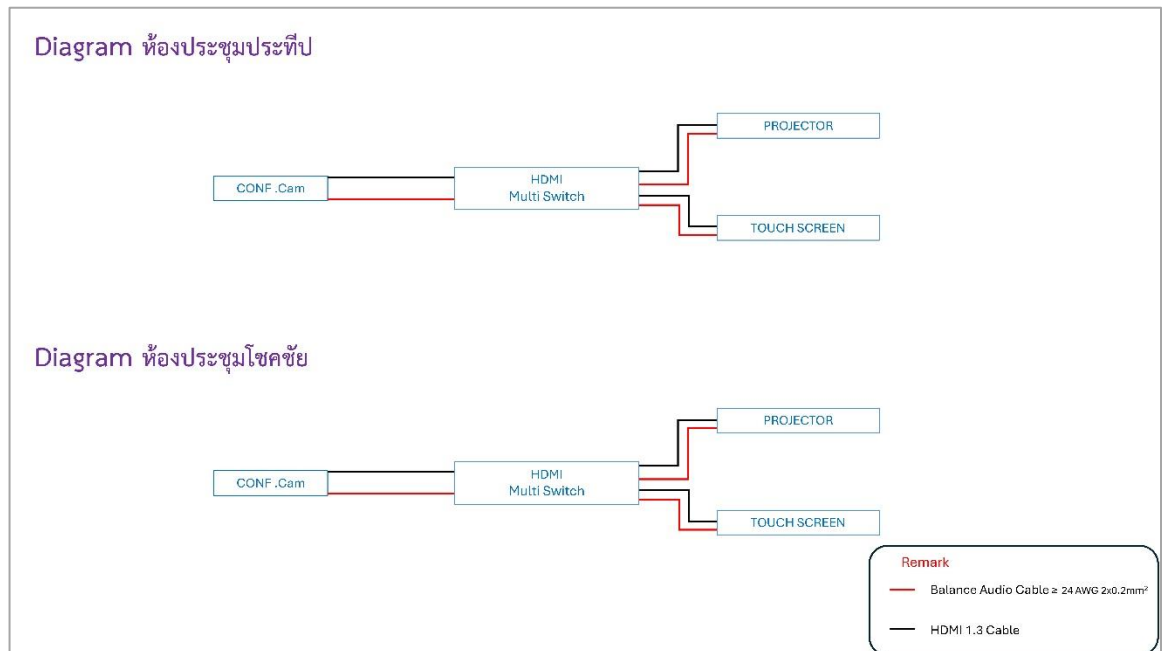
รูป 8.1 – ไดอะแกรมติดตั้งระบบภาพและเสียง ห้องประชุมประทีป/ ห้องประชุมโชคชัย
