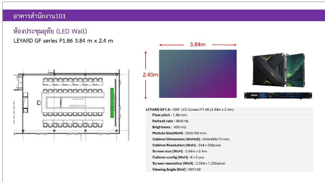
รูป 4.1 - แบบแปลนชั้น 2 อาคารสำนักงาน 101 แสดงตำแหน่งติดตั้งจอ LED ห้องประชุมอูทัย
