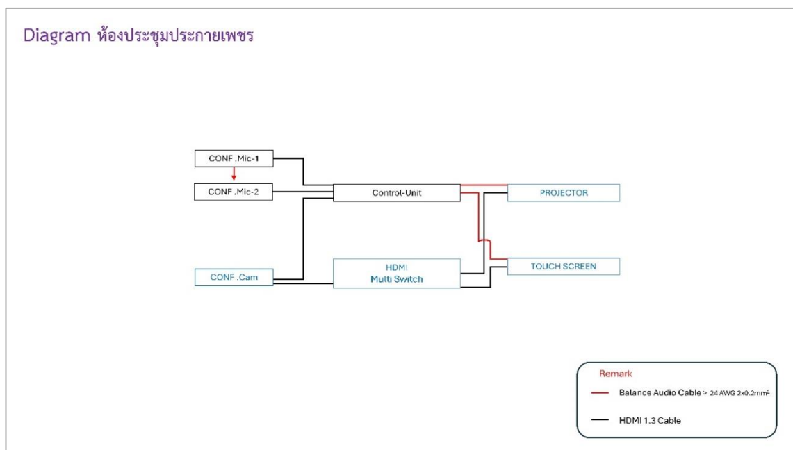
รูป 7.1 – ไดอะแกรมติดตั้งระบบภาพและเสียง ห้องประชุมประกายเพชร
