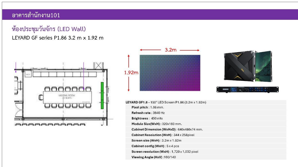
รูป 5.1 - แบบแปลนชั้น 2 อาคารสำนักงาน 101 แสดงตำแหน่งติดตั้งจอ LED ห้องประชุมวันจักร
